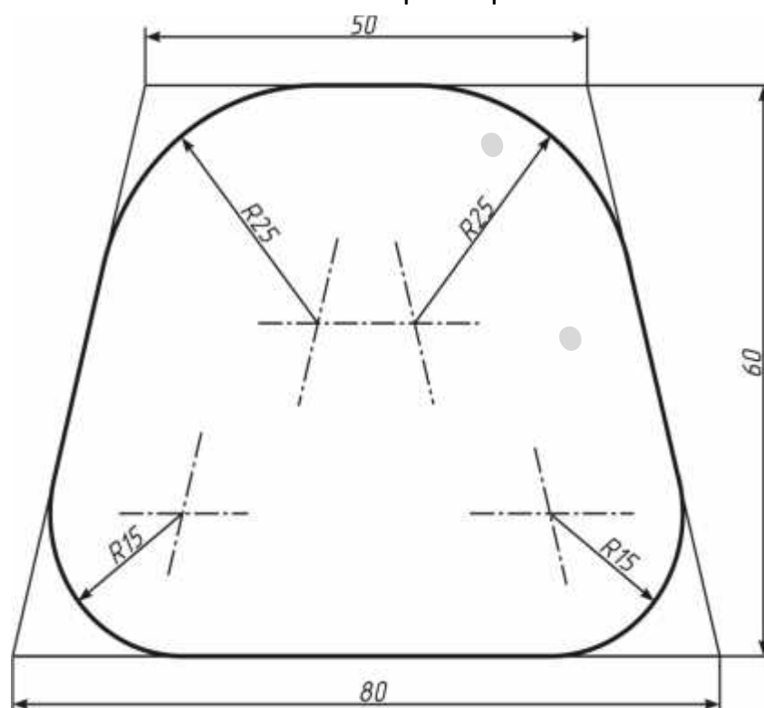
Нанесение размеров
